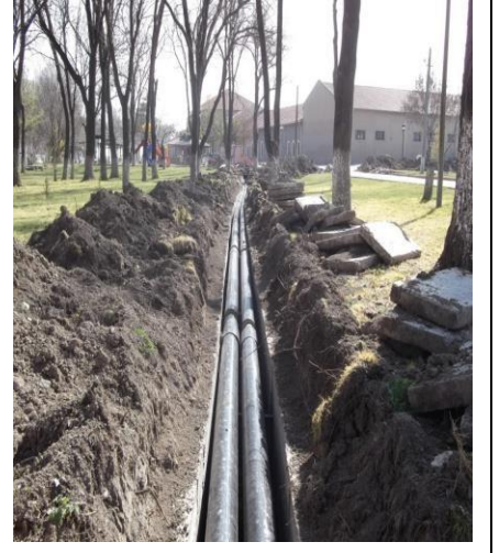
TİGEM ANADOLU TARIM İŞLETMESİ MÜDÜRLÜĞÜ MAHMUDİYE ISI HATLARININ YENİLENMESİ VE KAZAN DAİRESİ YAPIMI
