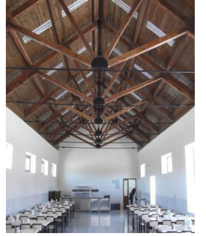
TİGEM ANADOLU TARIM İŞLETMESİ MÜDÜRLÜĞÜ MAHMUDİYE MUTFAK VE YEMEKHANE BİNASI
